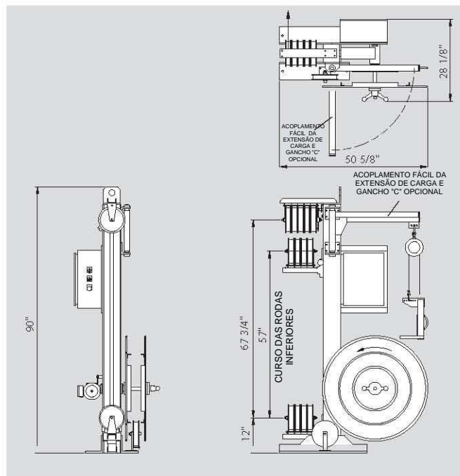
Desbobinador Jumbo para Fitas de Poliéster CD12
