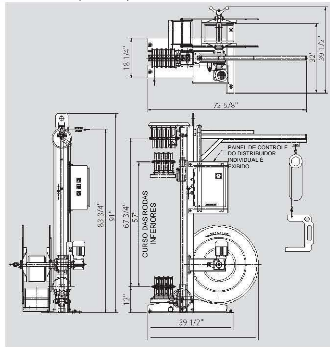
Desbobinador Super Jumbo para Fitas de Poliéster CD12SJ
